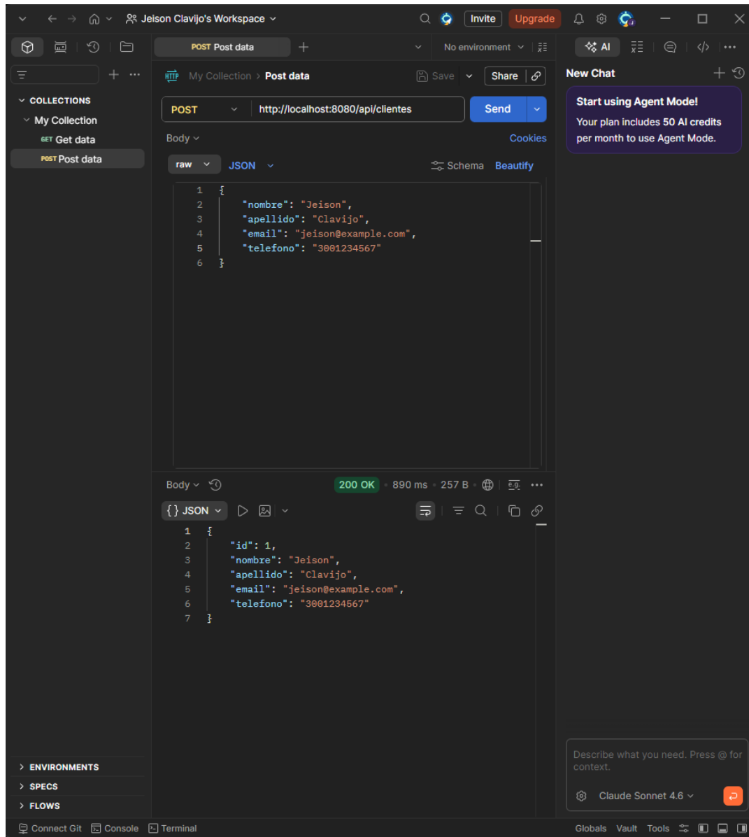
Ilustración 3. Prueba del método de crear clientes
