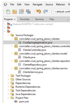
Ilustración 11. Evidencia de la estructura del proyecto
