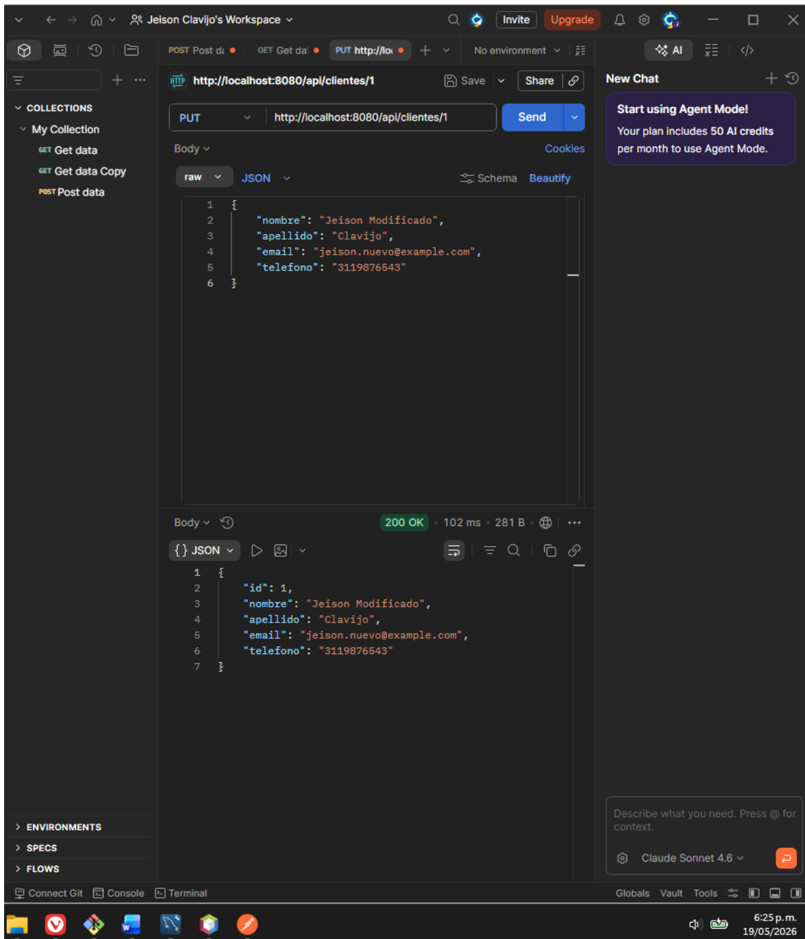
Ilustración 5. Prueba del método de modificar clientes
