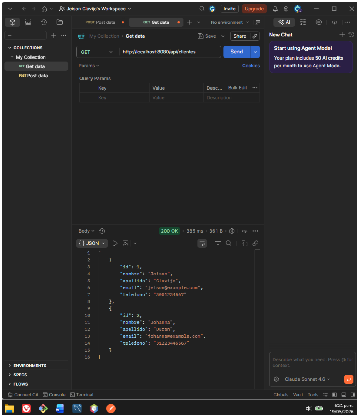
Ilustración 4. Prueba del método de consultar clientes
